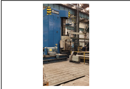
Plattenbohrwerk - Traghülse
